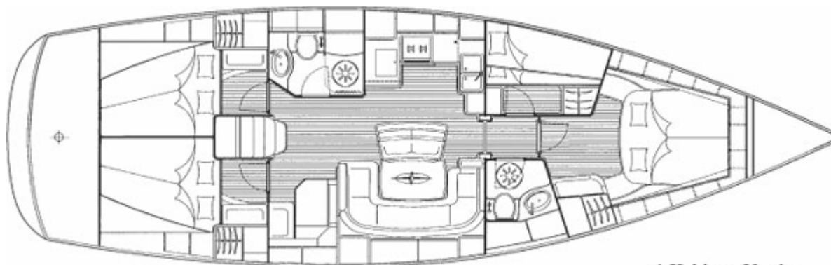
4-Kabinen-Version
